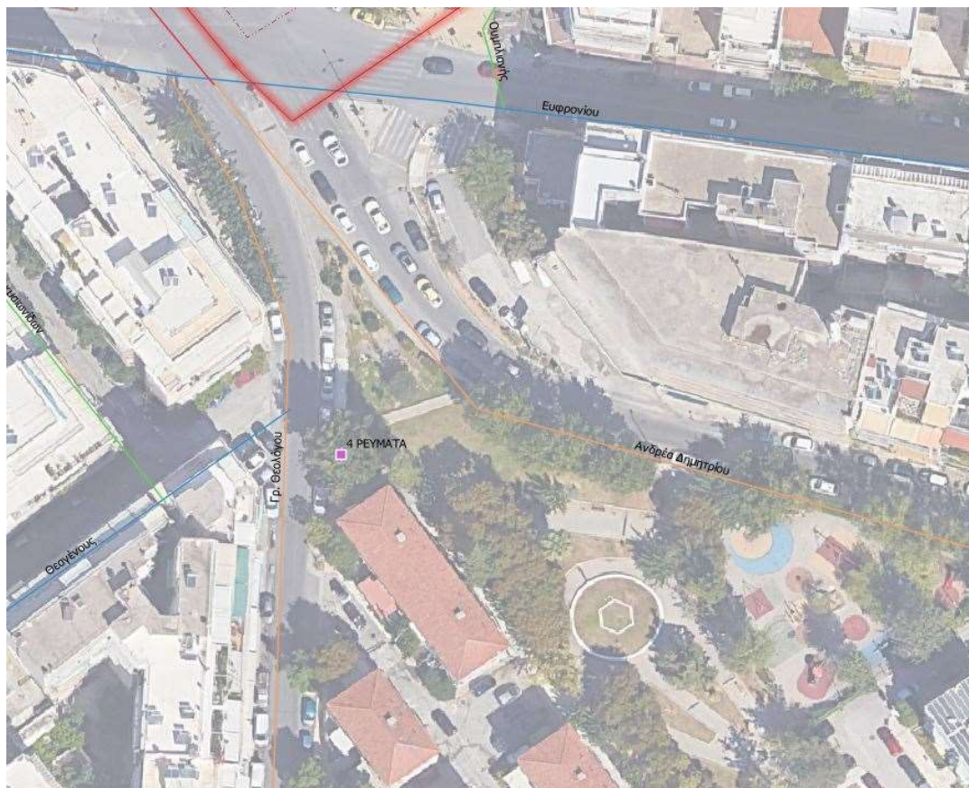
10) ΓΡ. ΘΕΟΛΟΓΟΥ υ ΔΗΜΗΤΡΙΟΥ (4 ΡΕΥΜΑΤΑ) 620mm X 220mm ΕΝΑΛΑΚΤΙΚΗ ΘΕΣΗ Α
